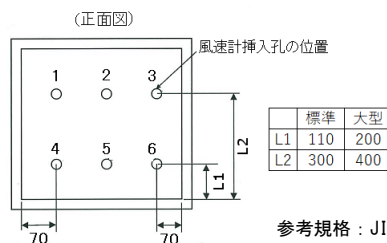
標準品の風速測定位置
